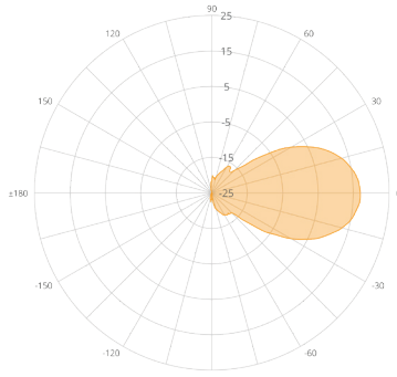
N5-X16 (16 dBi)
