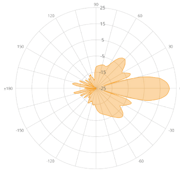
N5-X20 (20 dBi)
